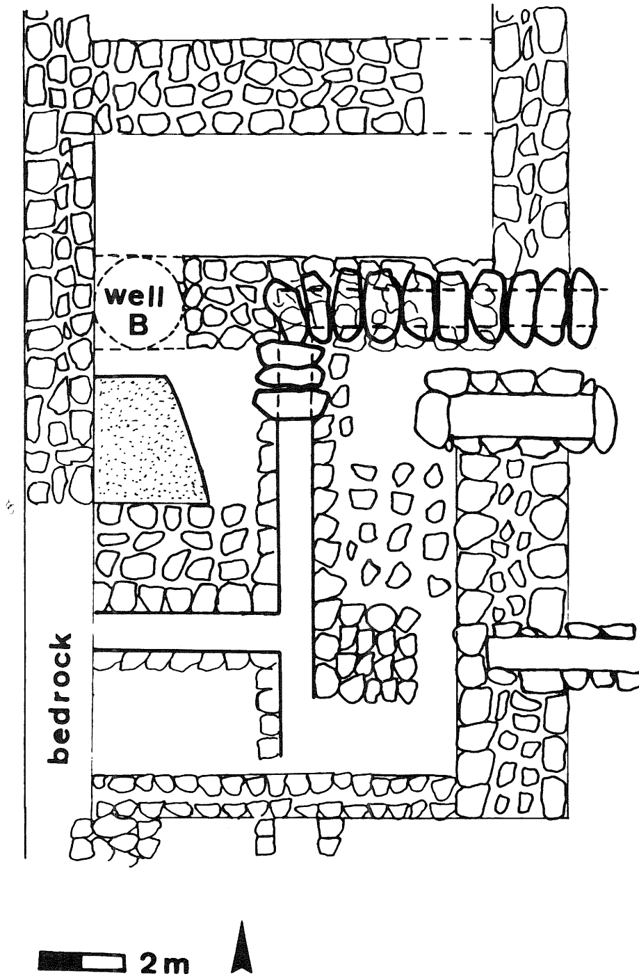
Εικ. 22. Μυκάναι, Δυτική Οικία, αποχετευτικός αγωγός, κάτοψις (ημερολόγιο ανασκαφεία).
