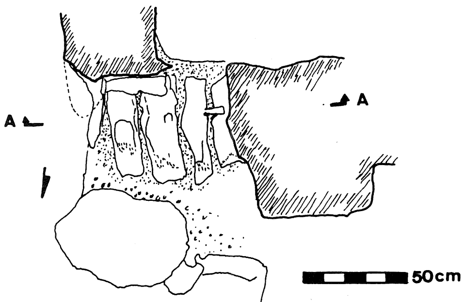
Εικ. 20. Μυκίνας, εστία Δυτικής Οικίας, κάτοψις, τομή (Βερδελής 1959, Εικ. 5).
