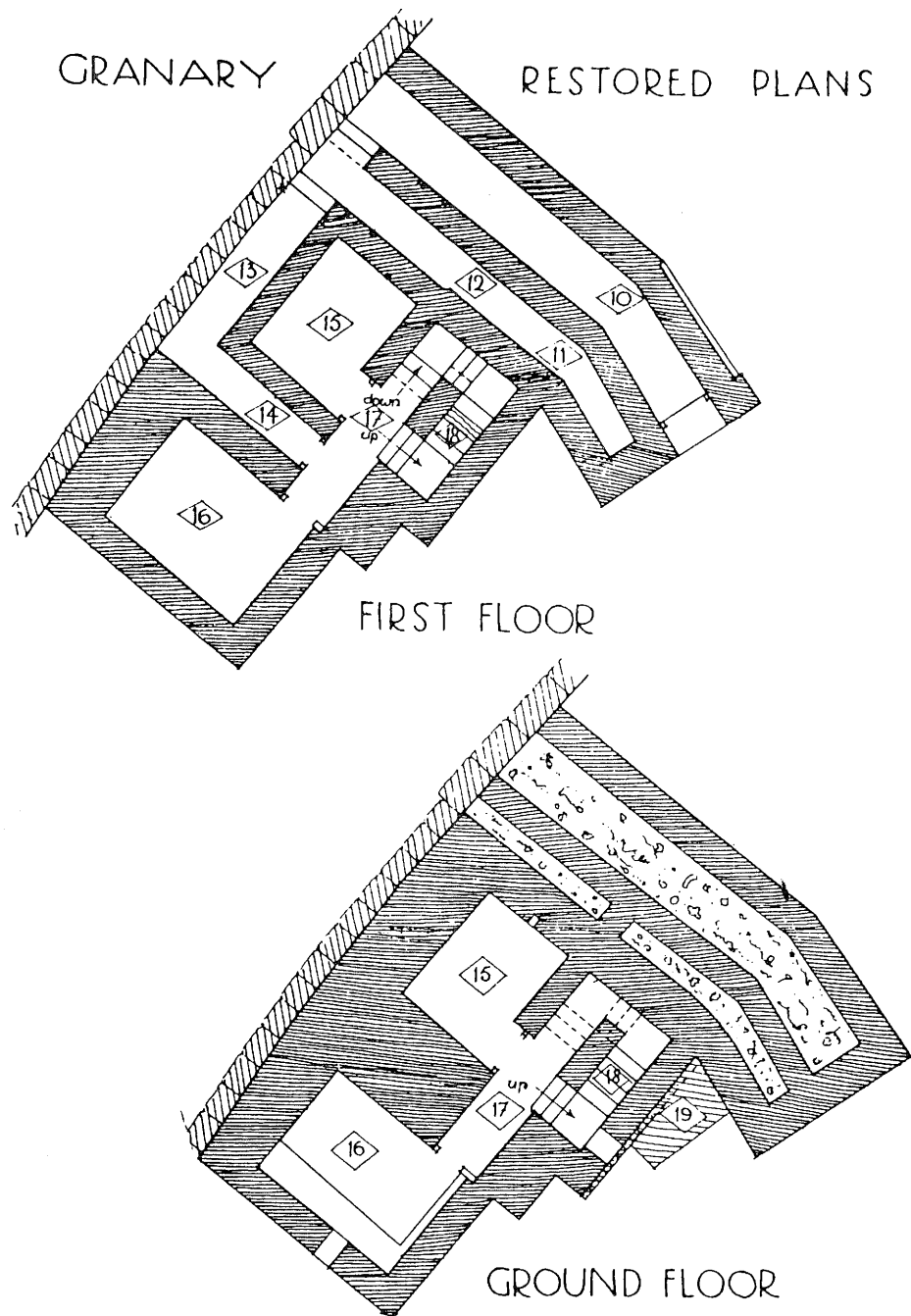
Εικ. 4. Μυκίνες, Σιταποθήκη, κάτοψις ισογείου (υπογείου) και πρώτου ορόφου (Wace 1949, Fig. 3).
