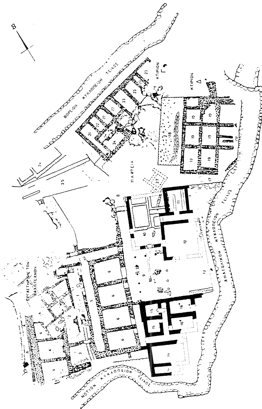
Εικ. 7. Μυκήναι, Οικία Κίωνων, Οικία Καλλιτεχνών (Ανατολική πτέρυγα του ανακτόρου (Ιακωβίδης 1977, Fig. 8).
