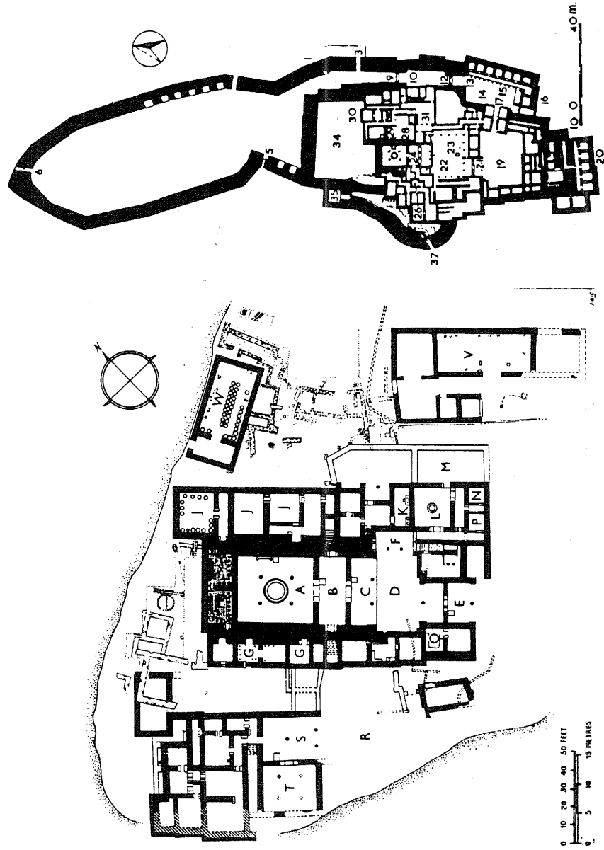
Εικ. 6. Κατόψεις ανακτόρων Πύλου και Τίφινθος (Taylor 1983, Fig. 75, 80).
