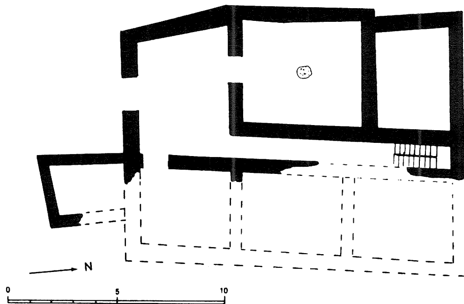
12. Μυκήναι, Οικία I λόφου Παναγίας (Mylonas-Shear 1987, Fig. 2).
