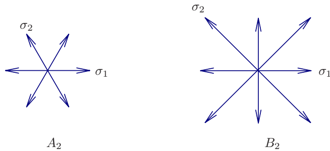
Σχήμα 1.2: Τα συστήματα ριζών των ομάδων A_2 και B_2 . Το πρώτο αντιστοιχεί στην ομάδα ανακλάσεων του ισοπλεύρου τριγώνου και το δεύτερο σε αυτήν του τετραγώνου.
