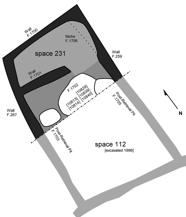
Εικόνα 68. Το κτήριο 50, Catalhöyük (Russell&Düring 2006, εικ. 2)
