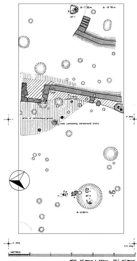
Εικόνα 60. Ύψη κατασκευών από τα στρώματα IX και X της Ακεραμικής Κνωσού (Reingruber 2001, εικ. 13)
